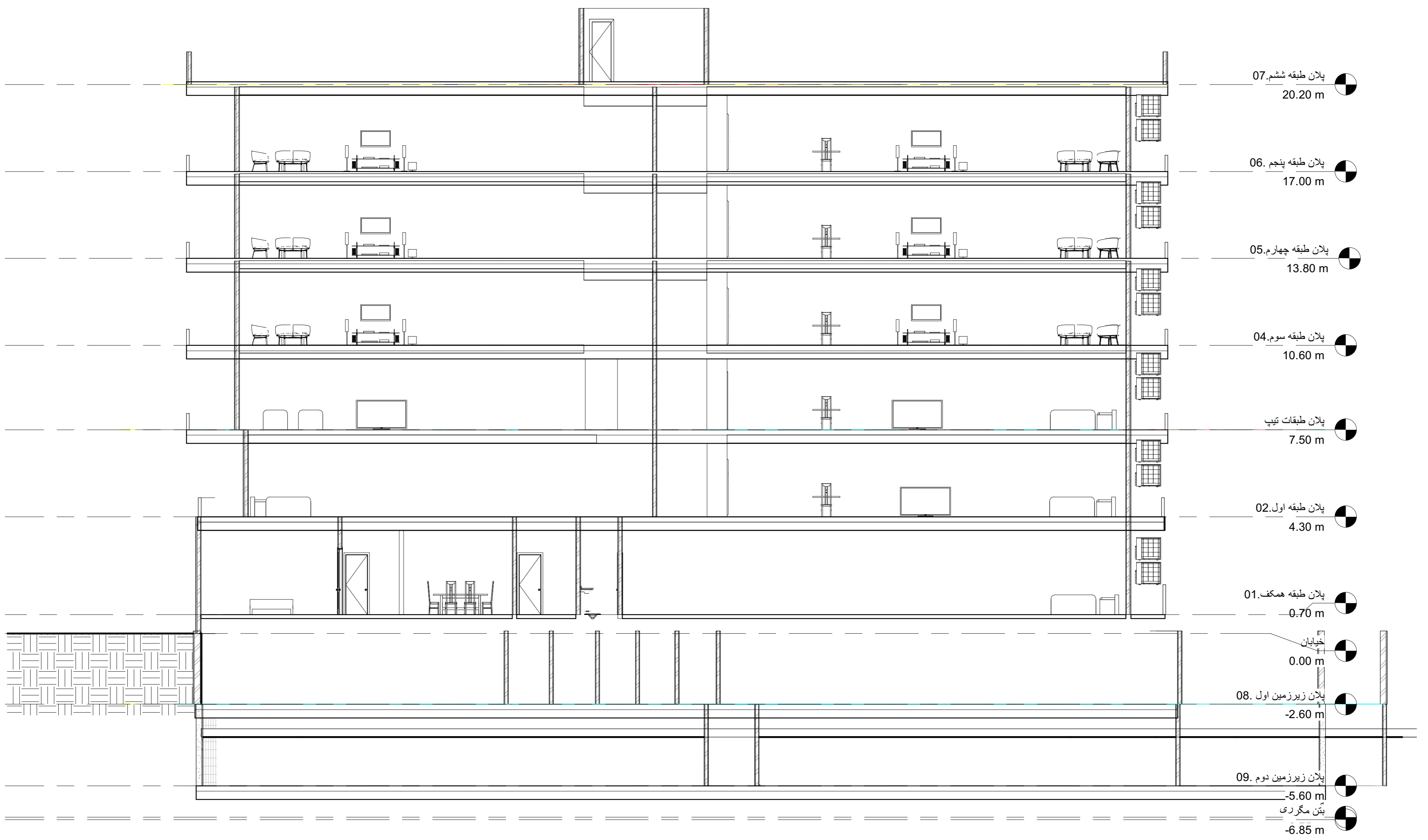
1 Section 1 1 : 100
